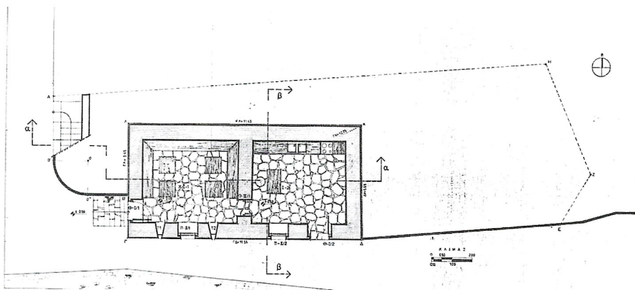
6. Σχέδιο Κατόψεως I επιπέδου (Μελέτη αποκαταστάσεως)
