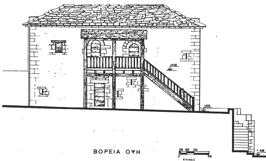
11. Σχέδιο Βορείας όψεως (Μελέτη αποκαταστάσεως)
