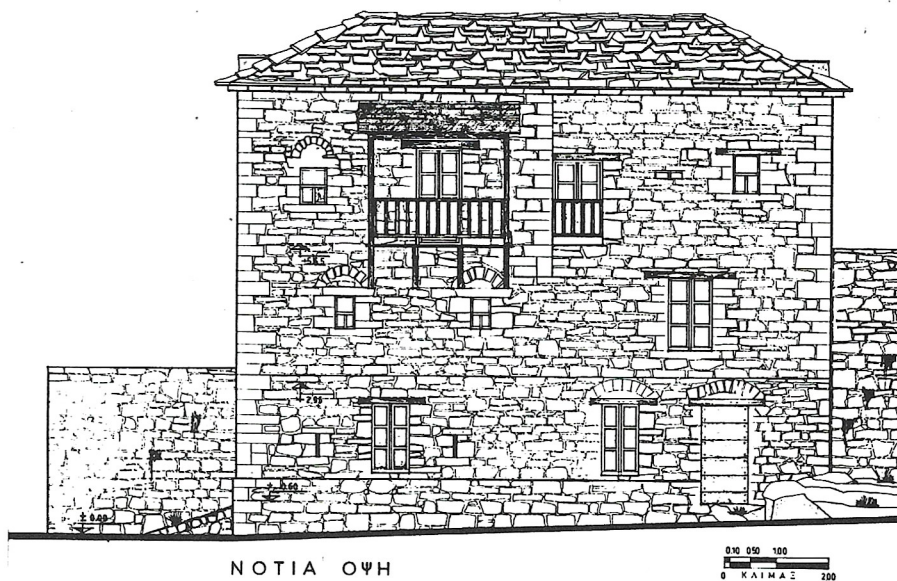
9. Σχέδιο Νοτίας όψεως (Μελέτη αποκαταστάσεως)
