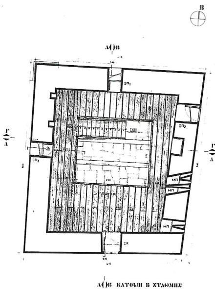
18. Σχέδιο κατόψεως Παταριού Ανατολικού Πύργου (Μελέτη αποκαταστάσεως)
