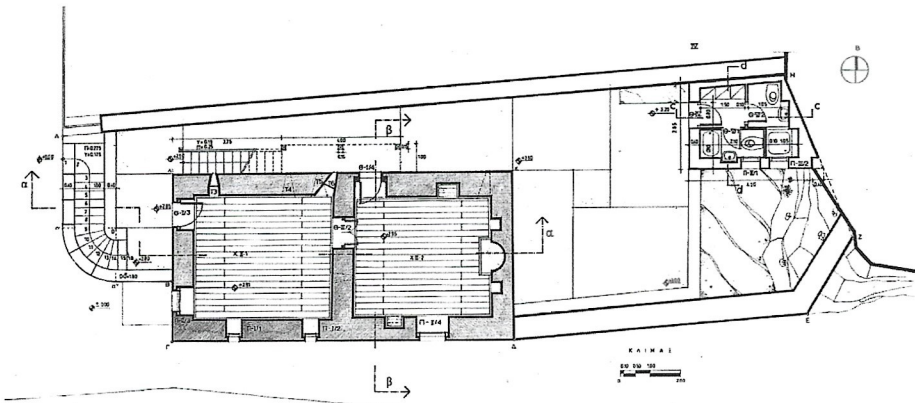
7. Σχέδιο Κατόψεως II επιπέδου (Μελέτη αποκαταστάσεως)
