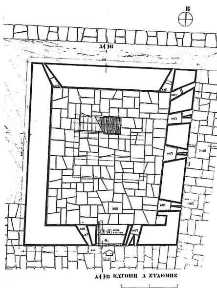
18. Σχέδιο κατόψεως Ανατολικού Πύργου (Μελέτη αποκαταστάσεως)
